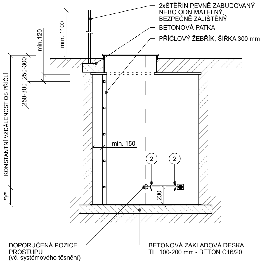
ŘEZ A-A'
