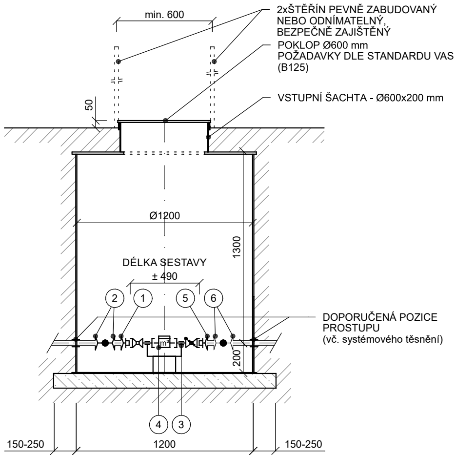
ŘEZ B-B'
